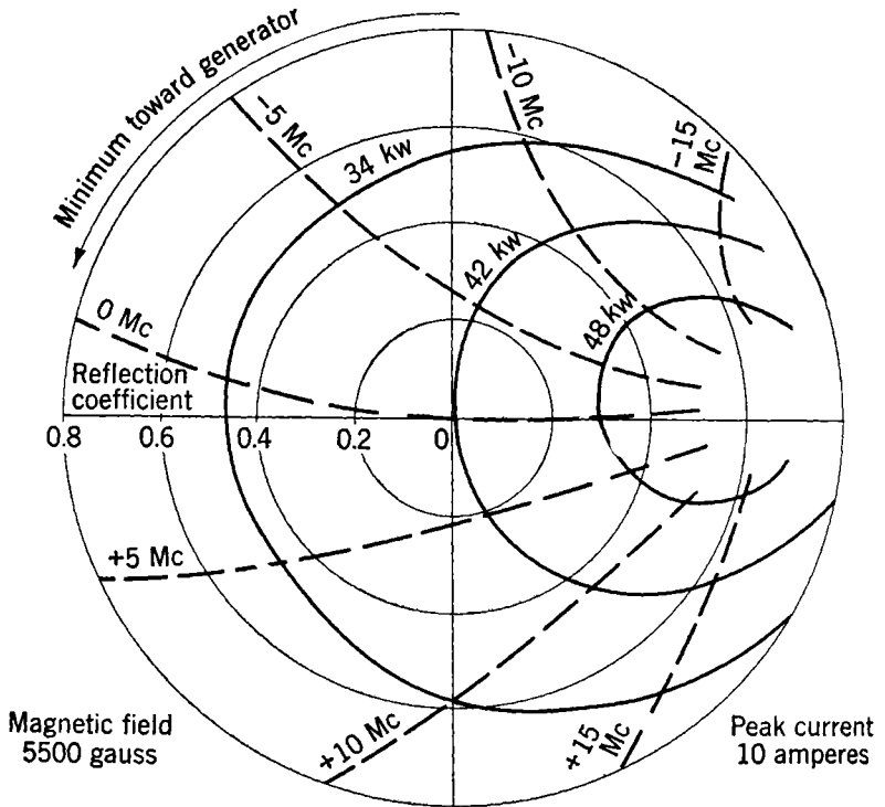
FIG. 19-45.—Rieke diagram for 725A magnetron.
